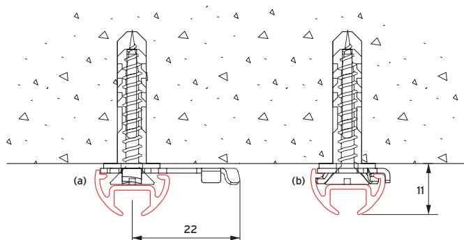
plafondmontage (2600) met spanner 2650 (incl. onderlegging 2649), voor (a) en na het aandraaien van de spanner (b): houdt 22mm vrij van de wand voor het draaien van de spanner
