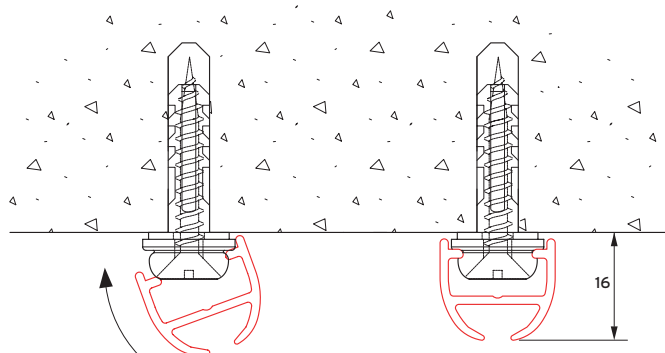
plafondmontage (2500) met clip 2254 en onderlegging 2649
