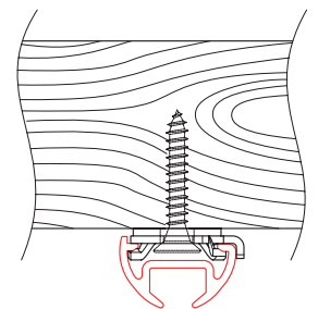
plafondmontage (2600) met spanner 2650, onderlegging 2649 en houtschroef 2614
